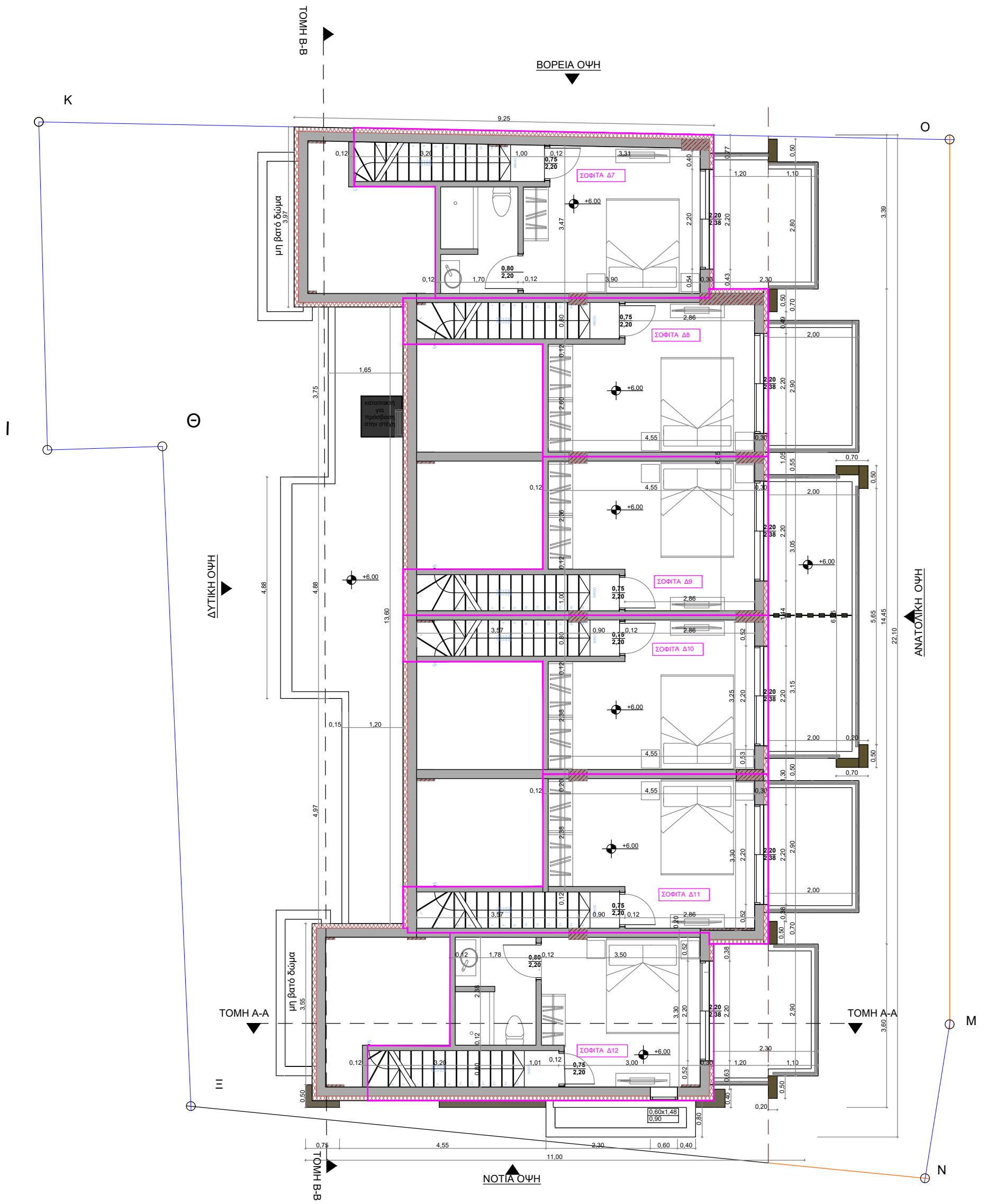
ΚΑΤΟΨΗ ΣΟΦΙΤΑΣ
